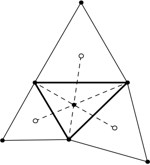
9.1) Napoleon point
